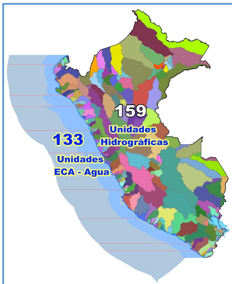
Figura N°01: “Unidades Hidrográficas en el Perú”
