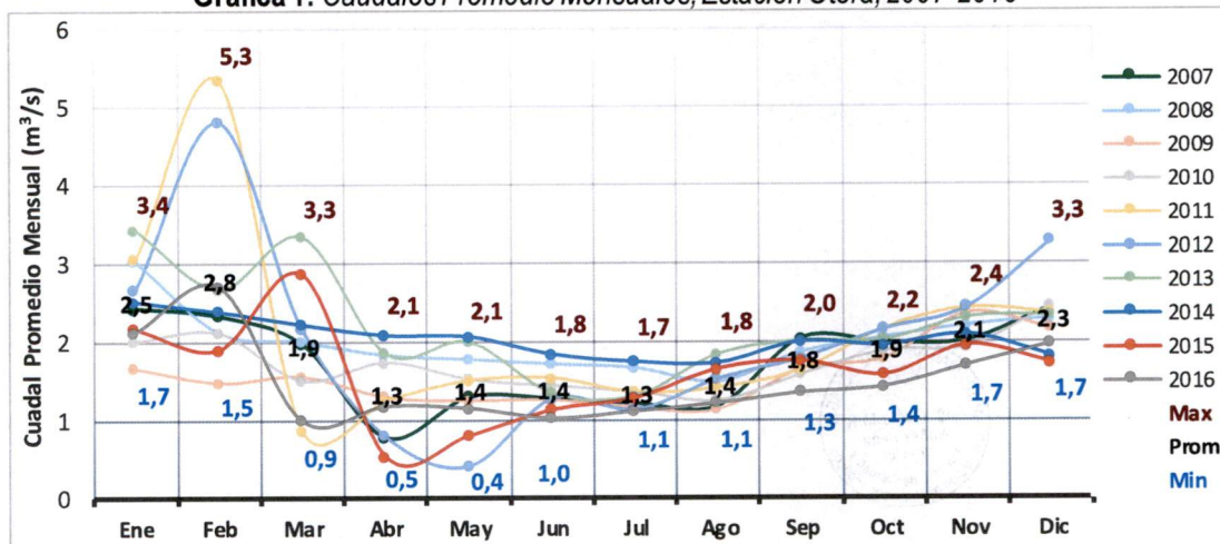
Gráfica 1: Caudales Promedio Mensuales, Estación Otor, 2007-2016
