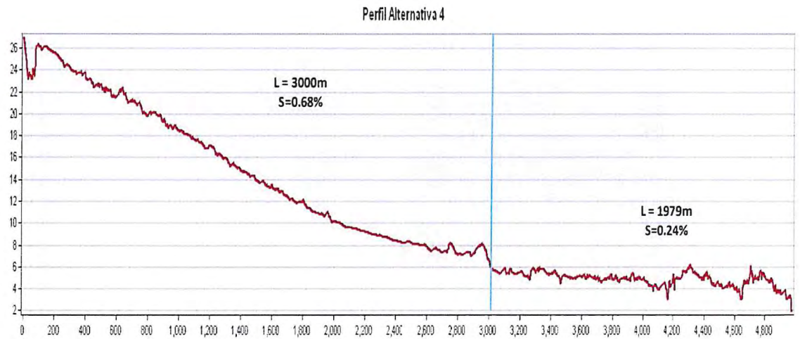
Gráfico 3: Perfil longitudinal de la ruta 4
