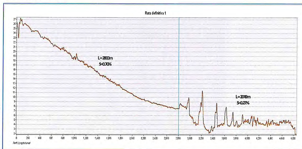
Figura N° 29: Perfil longitudinal de alternativa 1 propuesta.
