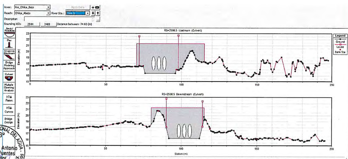
Figura N° 5: Alcantarilla en el cauce del río Chilca aguas abajo del partidor progresiva 2+506.5
