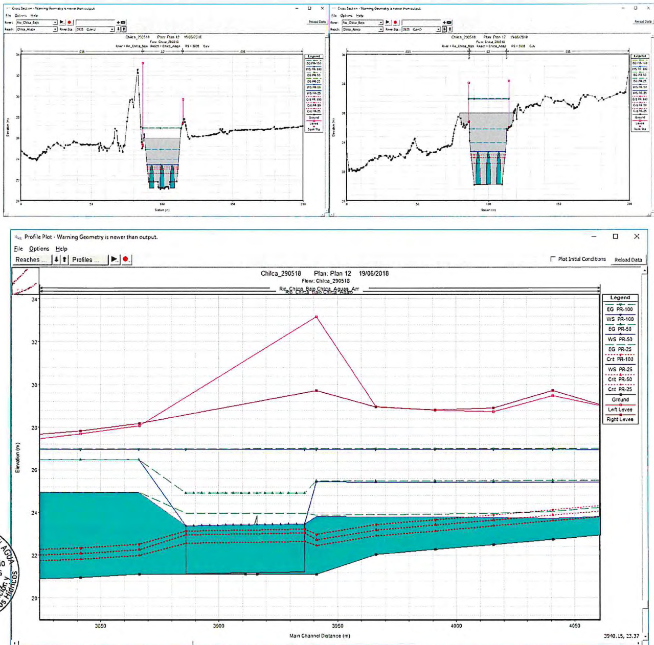
Figura N° 10: Resultados de HEC-RAS de la alcantarilla de la progresiva 3+935
