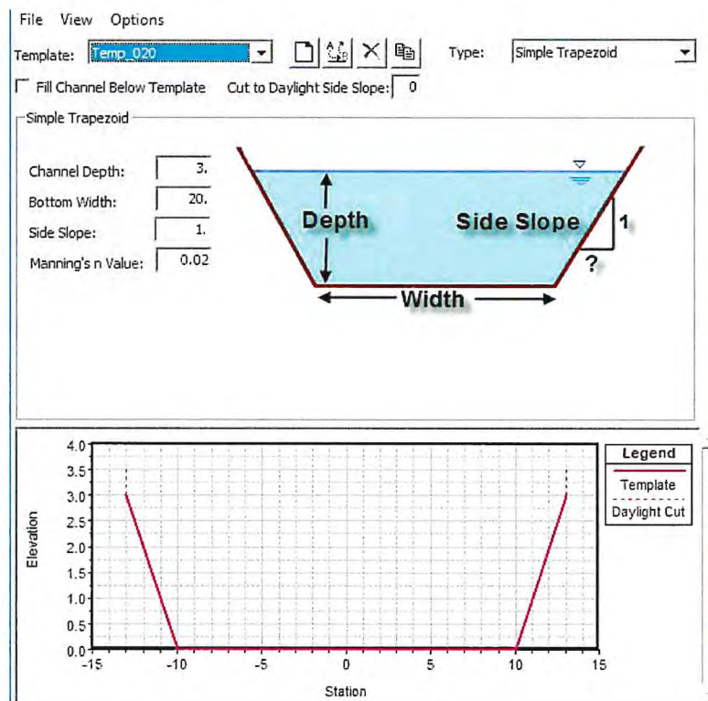
Gráfico N° 15: Sección propuesta en el cauce Sur del rio Chilca
