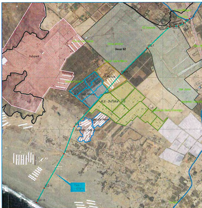
Figura N° 32: Ruta de descarga del CAUCE NORTE – alternativa 2.
