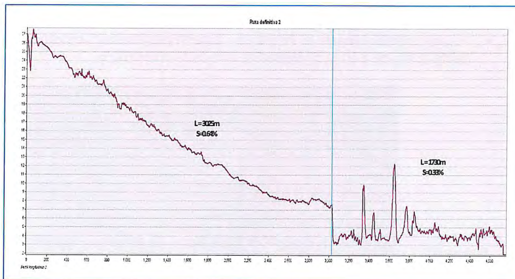
Figura N° 31: Perfil longitudinal de alternativa 2 propuesta.
