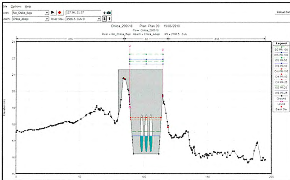
Gráfico 13: Resultados de HEC-RAS de la alcantarilla sobre cauce sur
