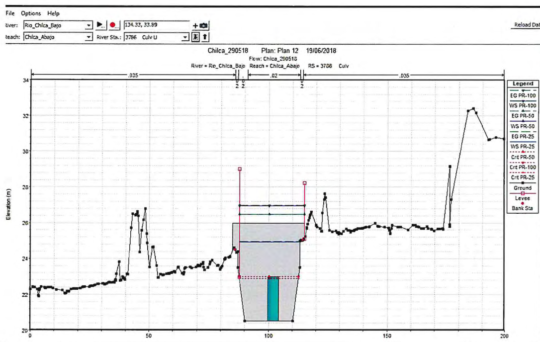
Gráfico 9: Resultados de HEC-RAS de la alcantarilla tipo cajón
