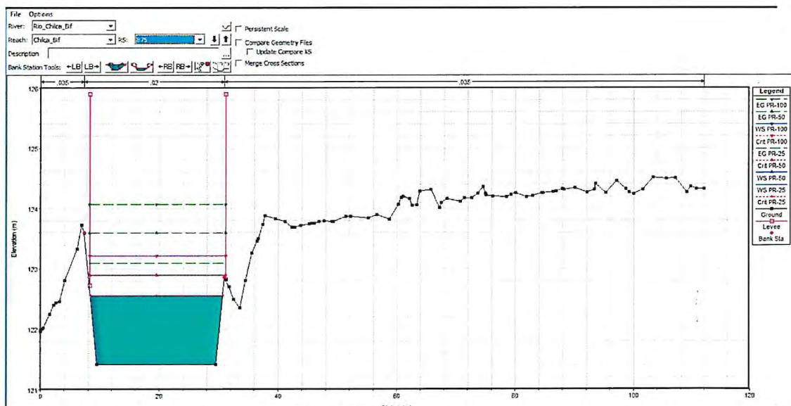
Grafico 6: Resultados de HEC-RAS, sección aguas abajo de partidor- cauce norte
