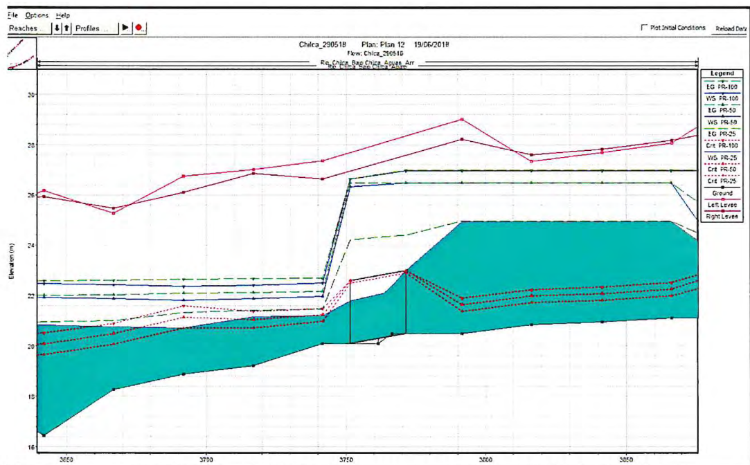
Gráfico 11: Resultados de HEC-RAS de la alcantarilla tipo cajón- perfil longitudinal
