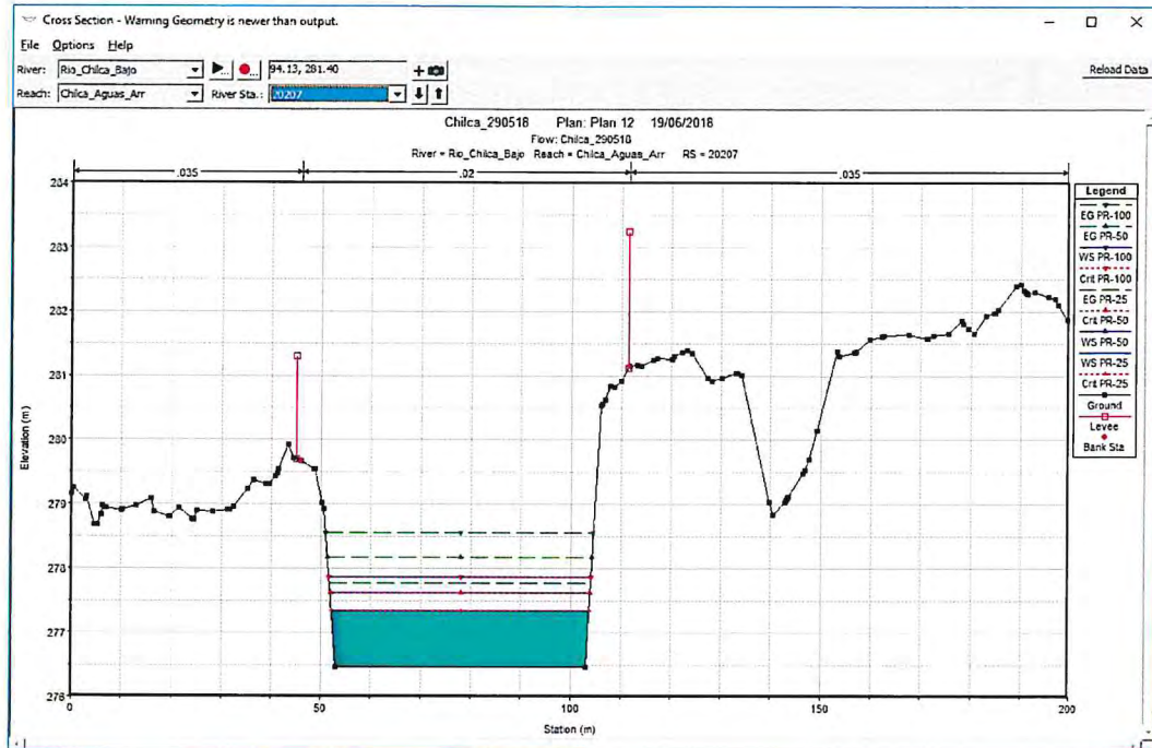
Figura N° 11: Sección propuesta en el cauce del río Chilca
