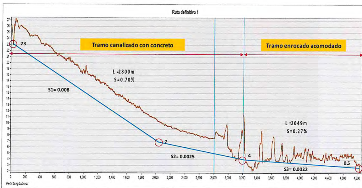
Gráfico N° 16: Perfil longitudinal de ruta de descarga-alternativa 1- cauce nor-oeste
