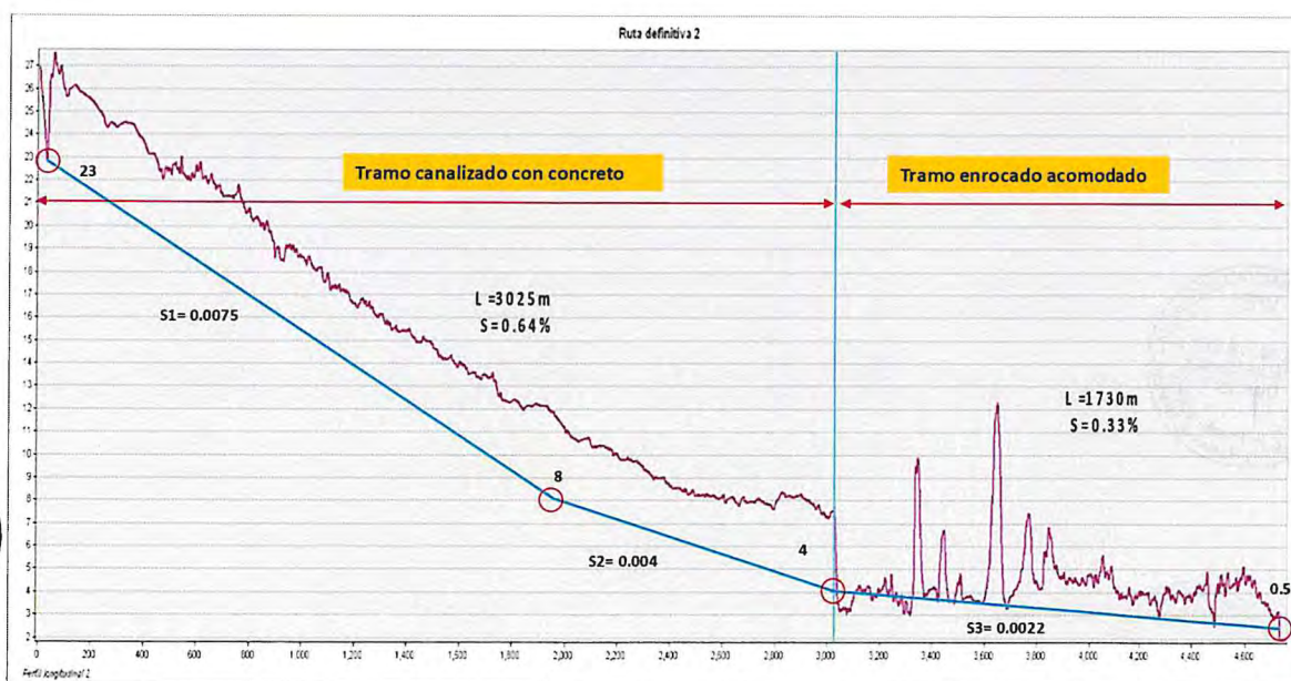
Gráfico N° 17: Perfil longitudinal de ruta de descarga-alternativa 2- cauce nor-oeste
