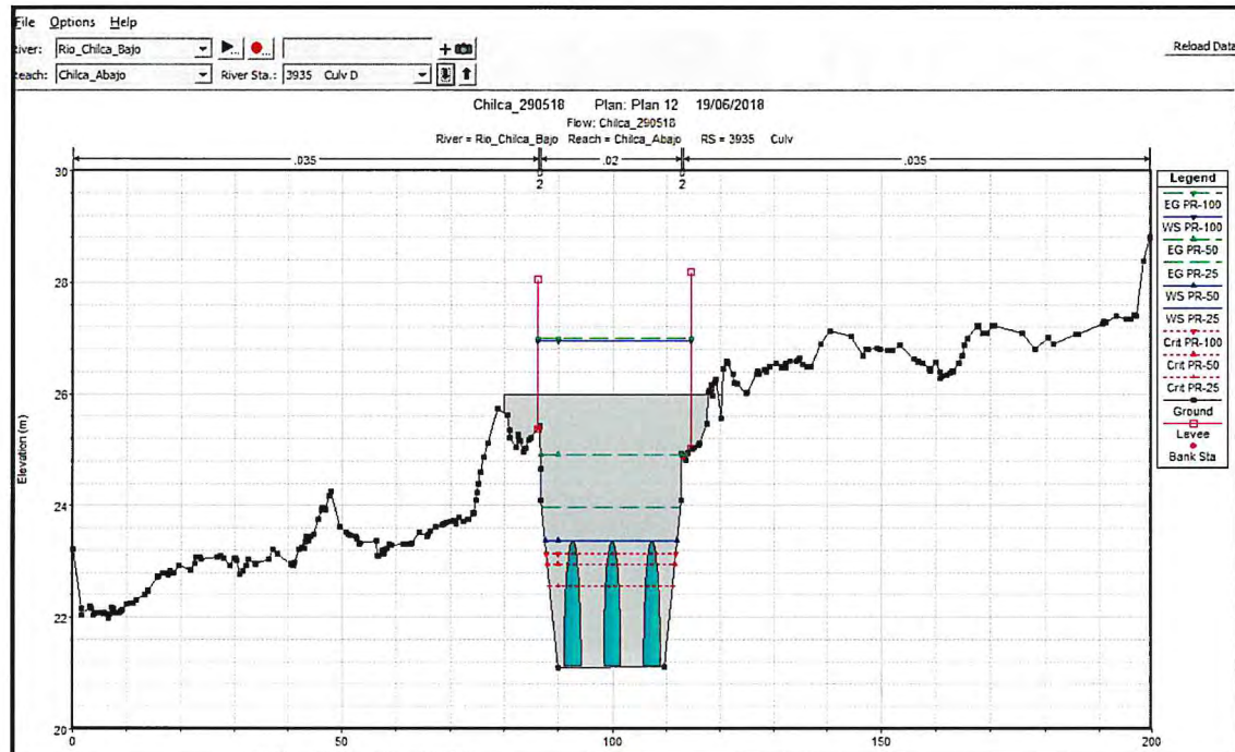
Gráfico 8: Resultados de HEC-RAS, sección de la alcantarilla sobre la panamericana sur
