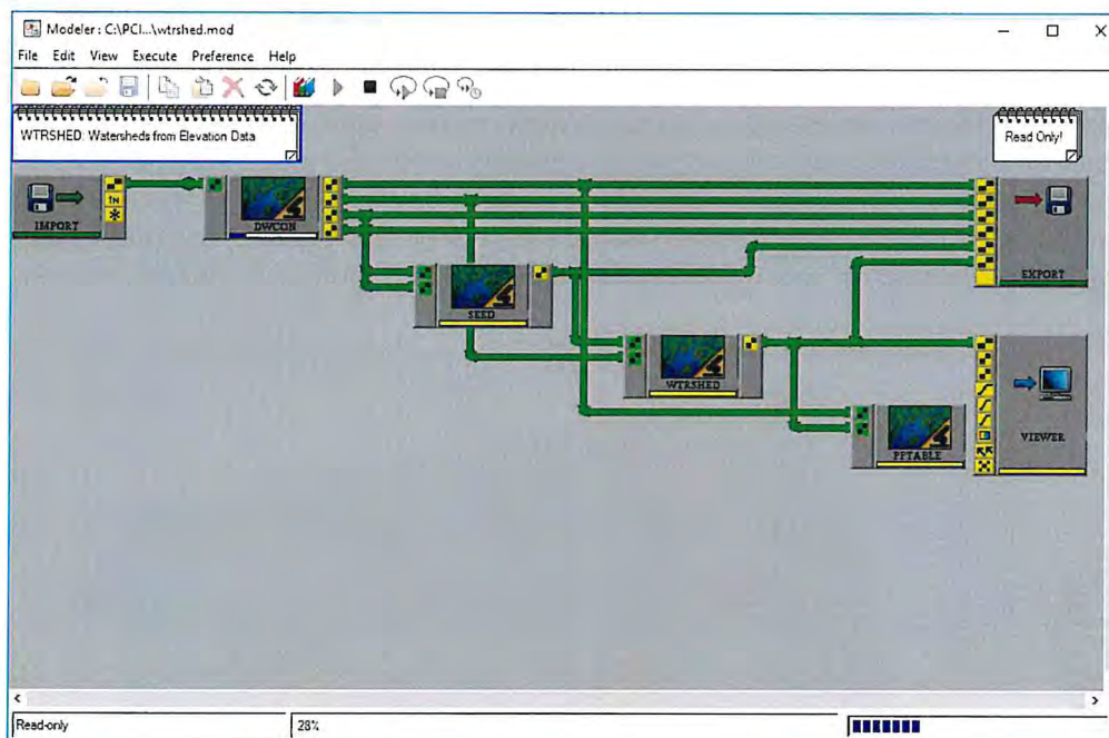
Figura N° 16: Flujo de trabajo para obtener cuenca colectora en el Modeler de PCI Geomatics 2017 SP1
