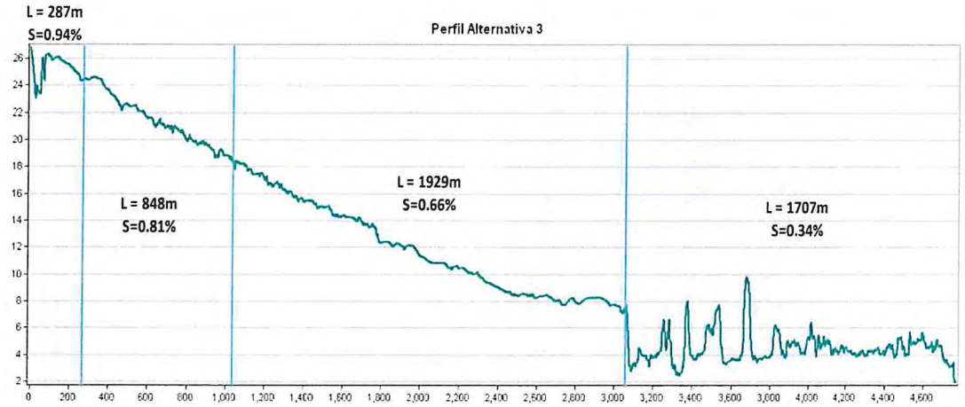
Gráfico 2: Perfil longitudinal de la ruta 3
