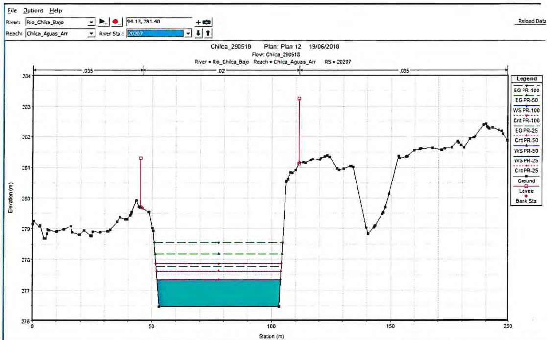
Gráfico 4: Resultados de HEC-RAS, sección aguas arriba de partidior
