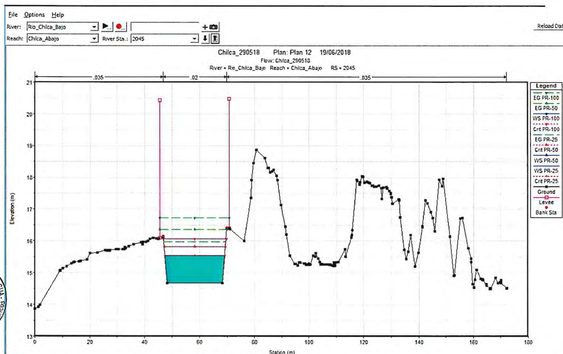
Grafico 5: Resultados de HEC-RAS, sección aguas abajo de partidor- cauce sur
