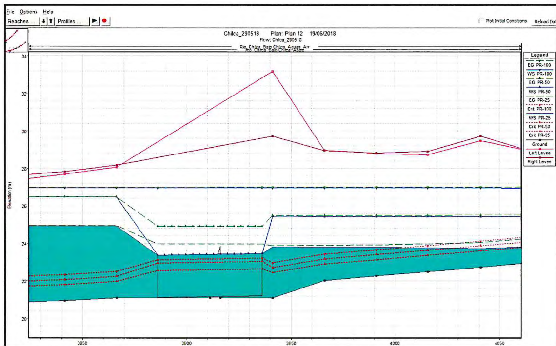
Gráfico 9: Resultados de HEC-RAS, perfil longitudinal de la alcantarilla sobre la panamericana sur
