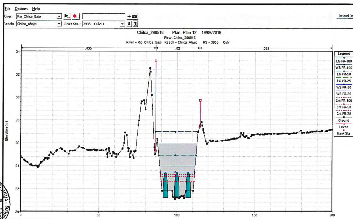
Grafico 7: Resultados de HEC-RAS, sección de la alcantarilla sobre la panamericana sur
