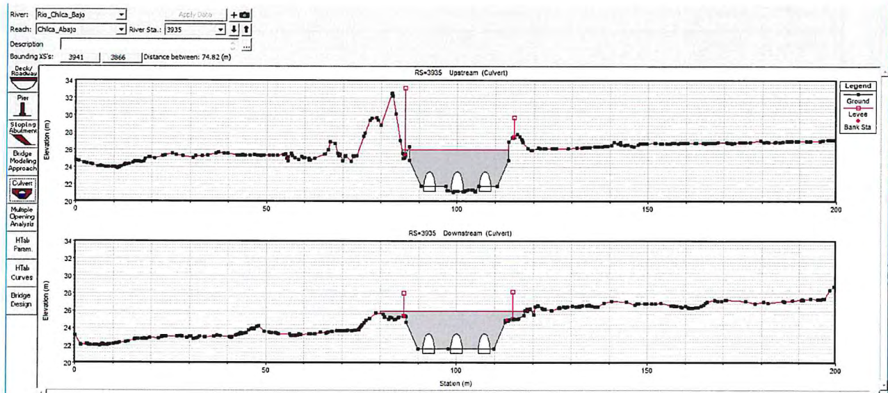
Figura N° 9: Alcantarilla en el cauce del rio Chilca aguas abajo del partidor progresiva 3+935
