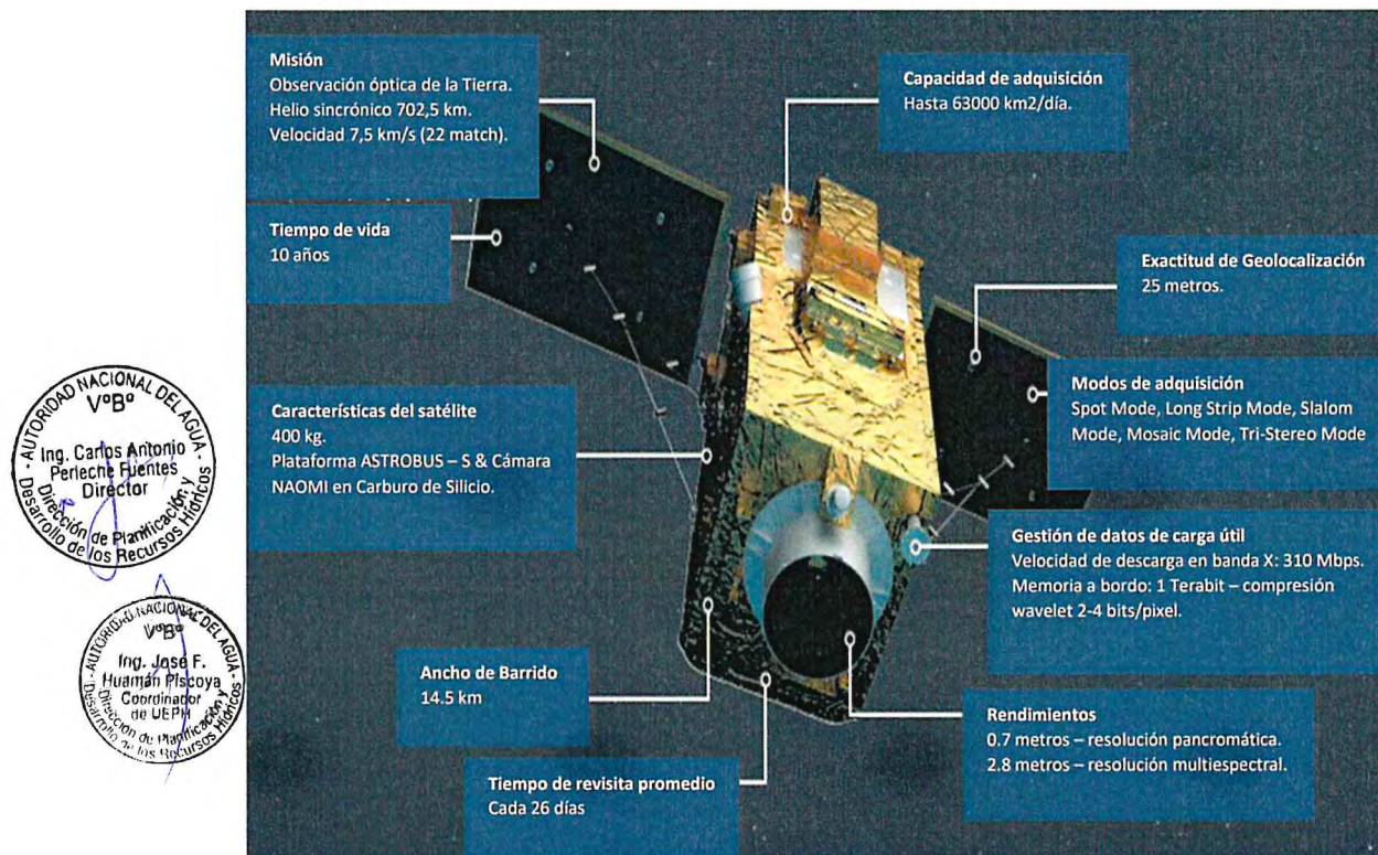
Figura N° 4: Representación del satélite peruano PeruSat-1. (Fuente: CONIDA).
