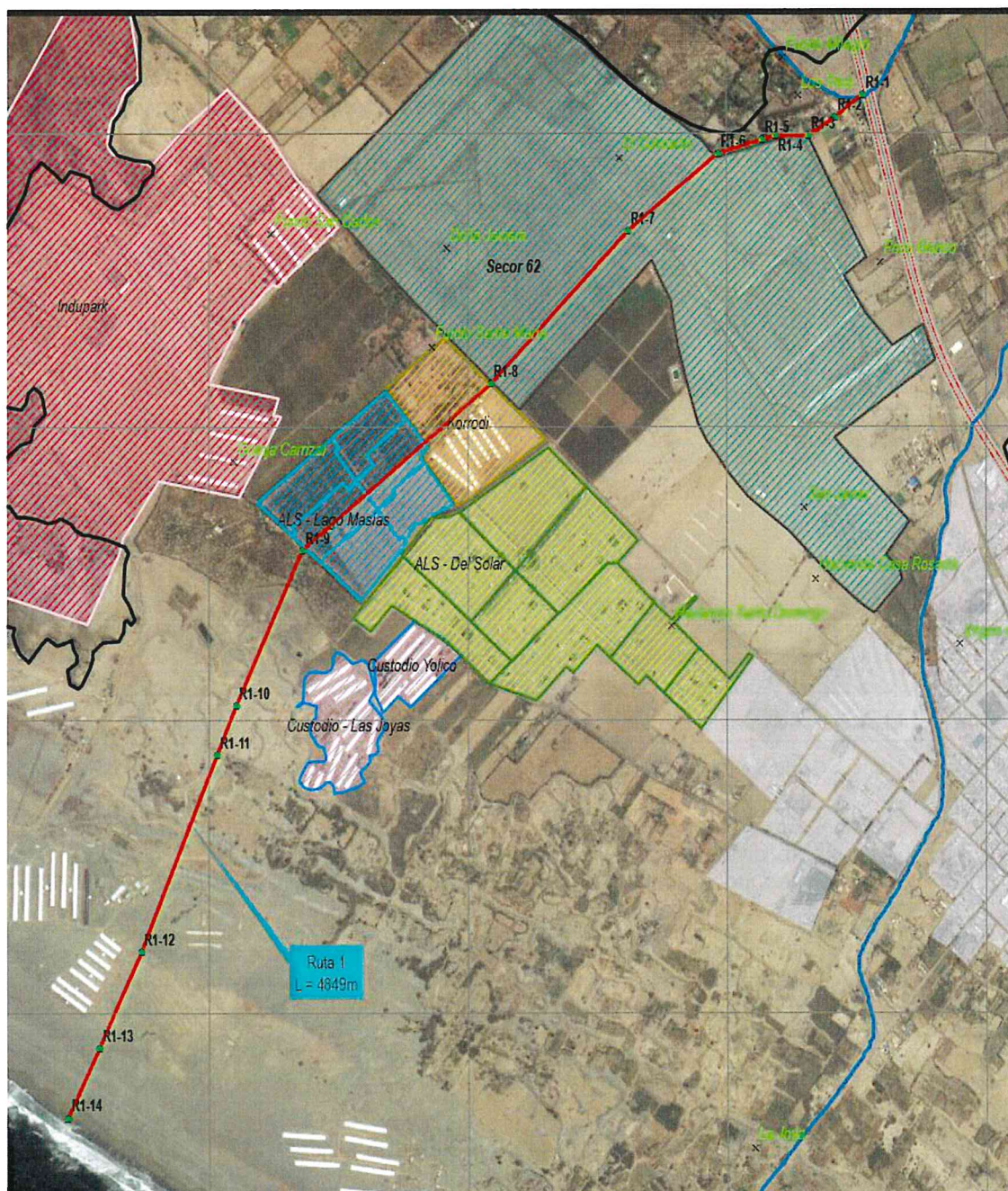
Imagen 18: Ruta de descarga del CAUCE HISTORICO NOR-OESTE – alternativa 1
