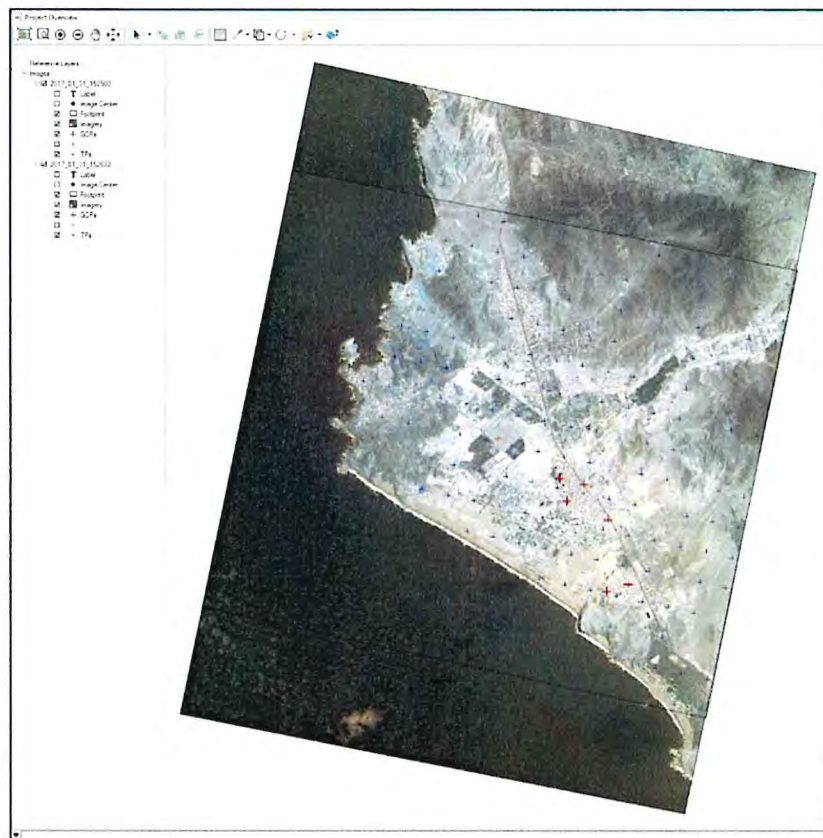
Figura N° 13: Visualización de los Tie Points (TPs) y Puntos de Control de Terreno (GCPs) en las dos escenas satelitales de PeruSat-1.
