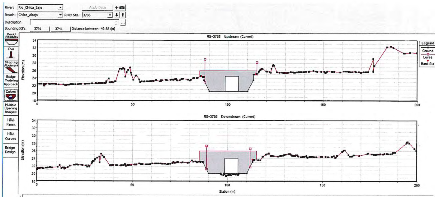
Figura N° 7: Alcantarilla en el cauce del rio Chilca aguas abajo del partidor progresiva 3+786
