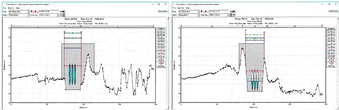
Figura N° 6: Resultados de HEC-RAS de la alcantarilla de la progresiva 2+506.5
