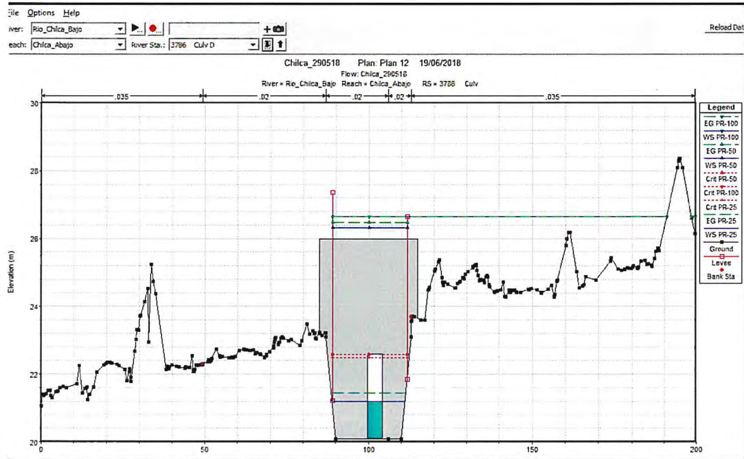
Gráfico 10: Resultados de HEC-RAS de la alcantarilla tipo cajón
