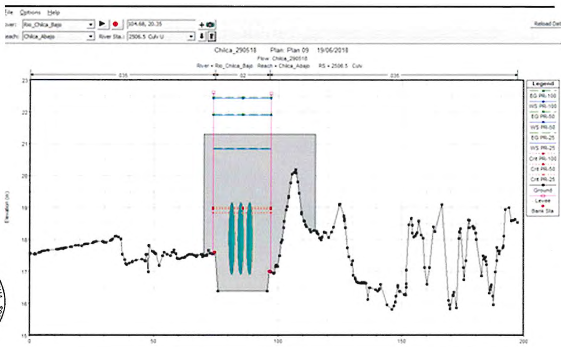
Grafico 12: Resultados de HEC-RAS de la alcantarilla sobre cauce sur
