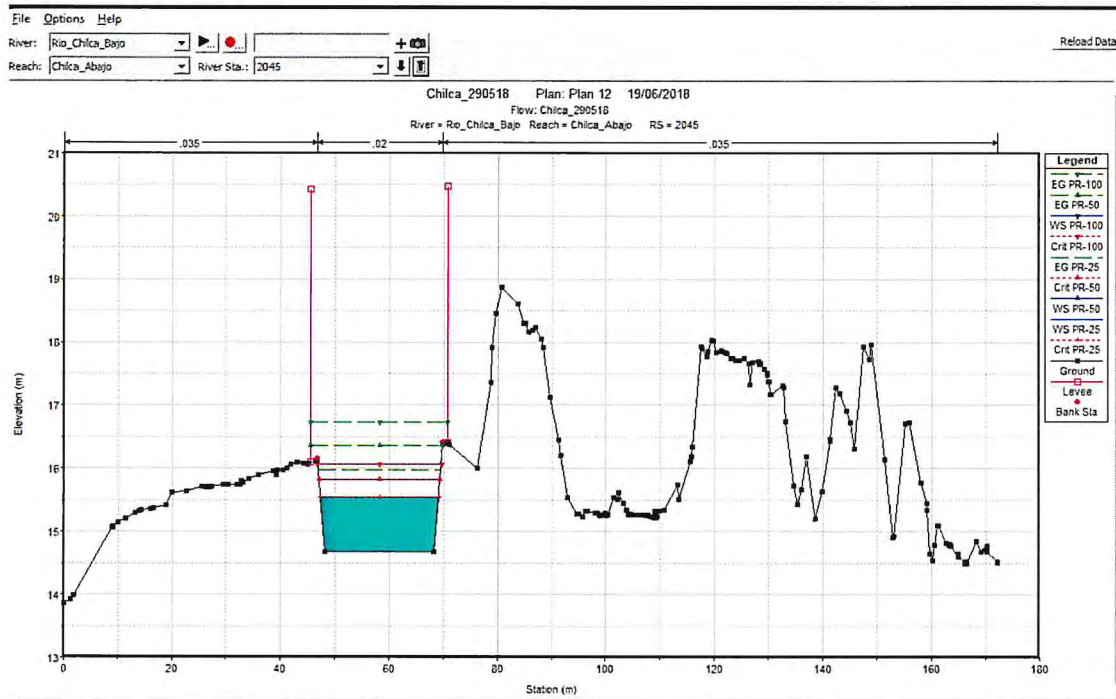
Gráfico N° 15: Sección propuesta en el cauce Sur del rio Chilca
