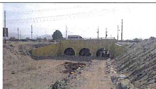
Foto 11: Vista aguas arriba del puente alcantarilla del llamado cauce norte.
