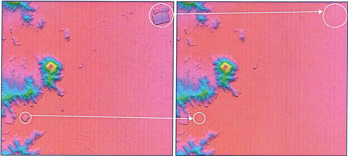
Figura N° 17: Resultado del filtrado del Modelo Digital de Superficie (DSM) a Modelo digital del Terreno (DTM) de la zona de estudio del satélite PeruSat-1
