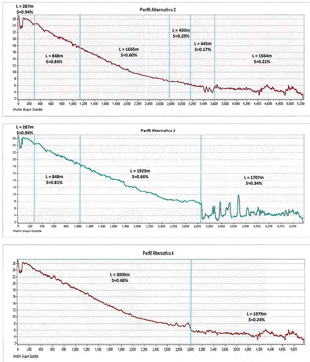
Figura N° 19: Perfiles topográficos de las tres alternativas de estudio planteadas para definir el cauce final del río Chilca.
