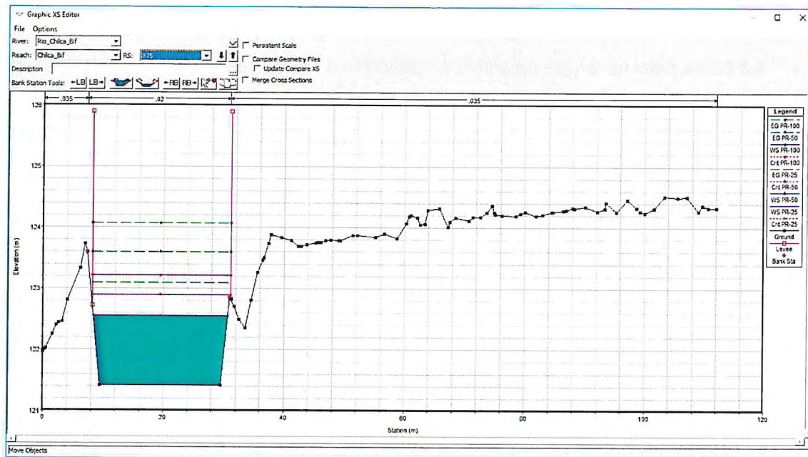
Figura N° 13: Sección propuesta en el cauce norte del rio Chilca
