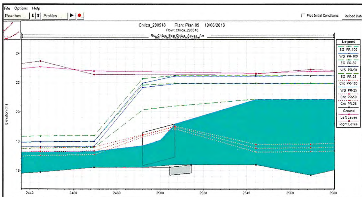
Gráfico 14: Resultados de HEC-RAS de la alcantarilla sobre cauce sur – perfil longitudinal
