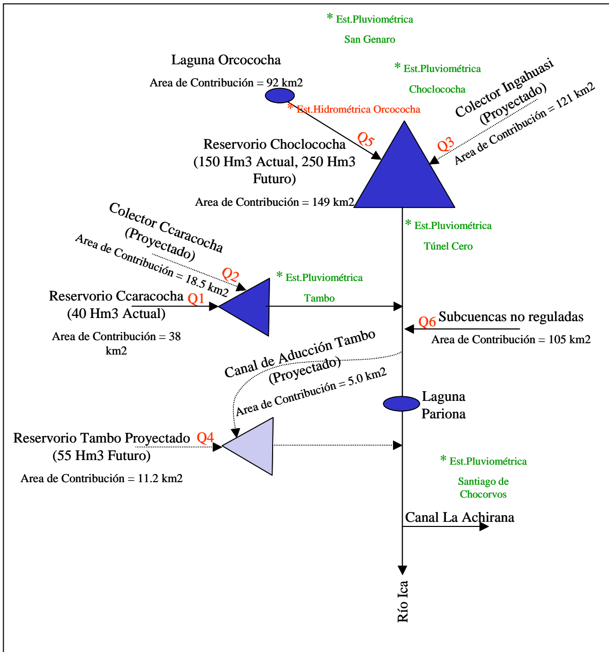
Figura N°02 Sistema Hidráulico Choclococha
